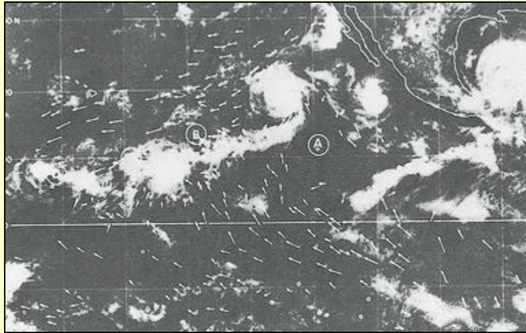
Պատկեր 17. Արբանյակային նկար, որը ցույց է տալիս ամպերը, որոնք շարժվում են միացման B,C, D տարածքներ: Սլաքները նշում են քամու ուղղությունը: (Արբանյակային Նկարների կիրառությունը Եղանակային Վերլուծության և Կանխատեսման համար, Անդերսոն և այլոք Էջ.188)
