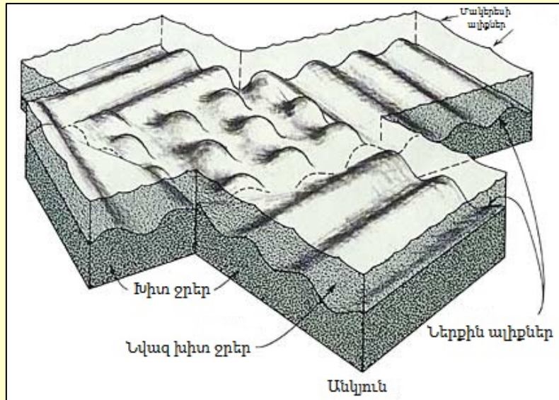
Պատկեր 16 Ներքին ալիքները ջրի տարբեր խտության երկու շերտերի մակերեսին: Մեկը խիտ է, ստորին ալիքը, մյուսը՝ նվազ խիտ, որը հանդիսանում է վերին ալիքը: (Օվկիանոսագիտություն Գրոսս Էջ.204)
