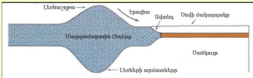
Պատկեր 9. Մեկ այլ լուսանկար ցույց է տալիս, թե լեռները ինչպես ցցանման են, ի շնորհիվ իրենց խորը արմատների: (Երկրագիտություն Թարրուք և Լուրգենս էջ.158)
