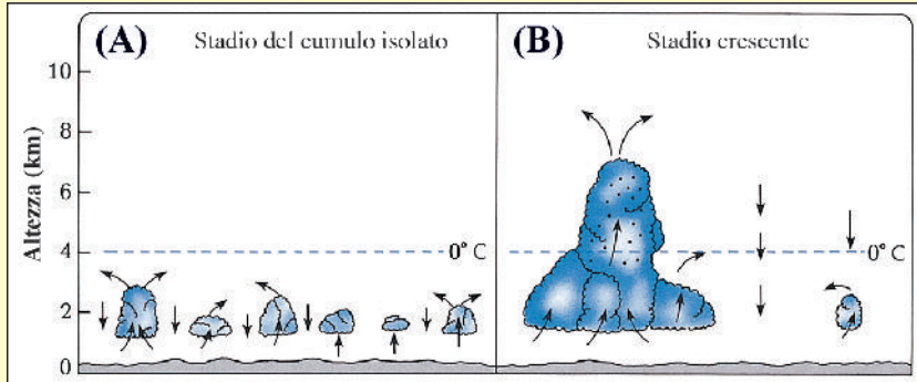
Figura 19: (A) Piccole nubi isolate (nubi cumulo). (B) Quando le piccole nubi si uniscono, le correnti ascensionali all'interno della grossa nube aumentano, così la nuvola si ingrandisce. Le gocce di pioggia sono indicate con \cdot . ( The Atmosphere (Atmosfera), Anthes e altri, p. 269.)
