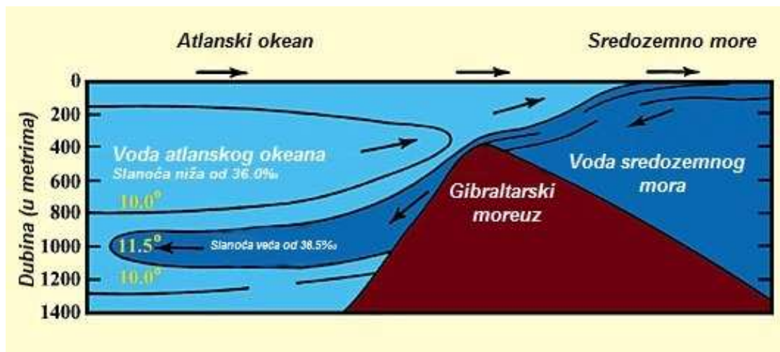
Slika 13: Vode Sredozemnog mora ulaze u Atlantski okean zadržavajući svoju temperaturu, slanoću i gustinu zbog pregrade između njih. (temperature su u stepenima celzijusa)
