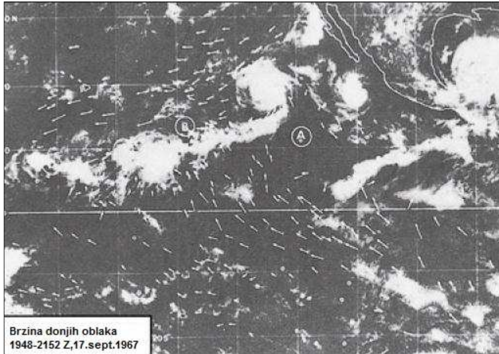
Slika 17: Satelitska slika pokazuje kretanje oblaka prema mjestu spajanja B, C i D. Strelice pokazuju pravac kretanja vjetra. ("Korištenje satelitskih slika u vremenskim analizama i prognozama", Anderson i drugi, str.188)
