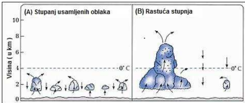
Slika 19(A): Odvojeni mali dijelovi oblaka (kumulusta).
