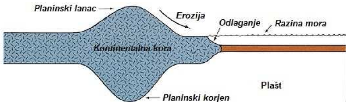
Slika 9: Slika pokazuje sličnost planina sa stubovima, zbog dubokog korjenja koje posjeduju. (Geologija, str. 158)
