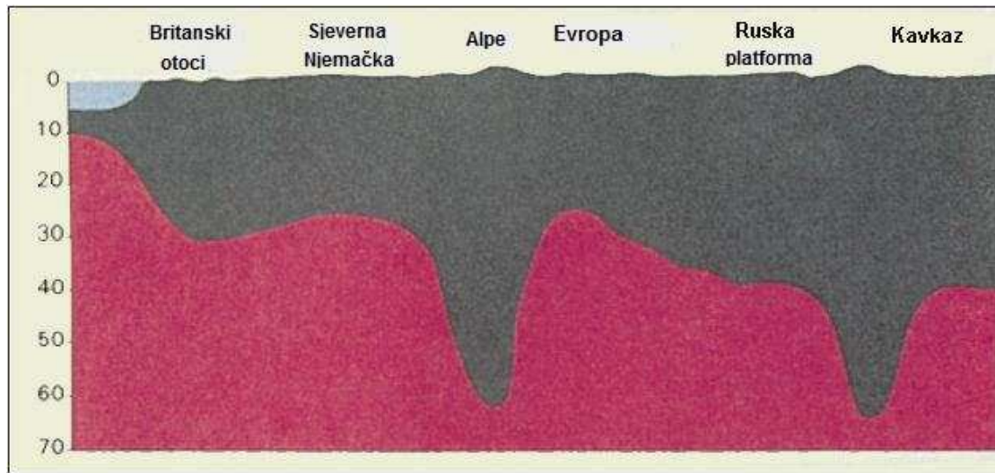
Slika 8: Šematski prikaz: Planine izgledaju poput stubova, imaju korjenje duboko u zemlji. (Anatomija Zemlje, str. 220)
