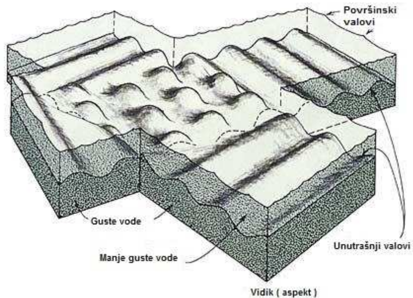
Slika 16: Unutrašnji valovi između sloja vode različitih gustina (jedna je gusta-donja, a druga manje gusta-gornja). Oceanography str.204
