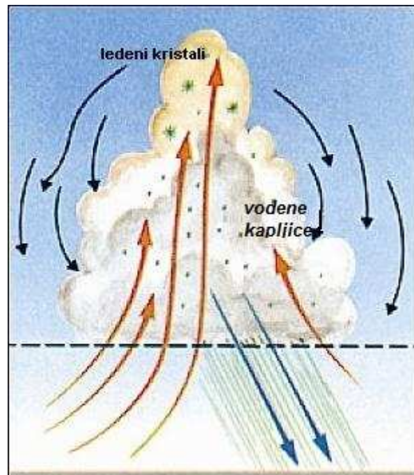
Slika 20: Kumulust. Nakon nagomilavanja oblaka počinje da pada kiša iz njega. (Vrijeme i klima, Bodin str.123)
